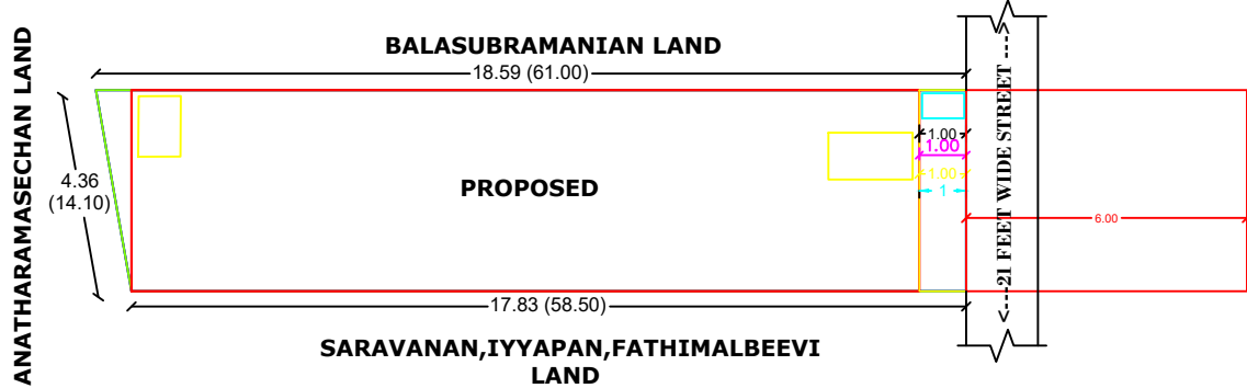
SITE PLAN SCALE 1:100
