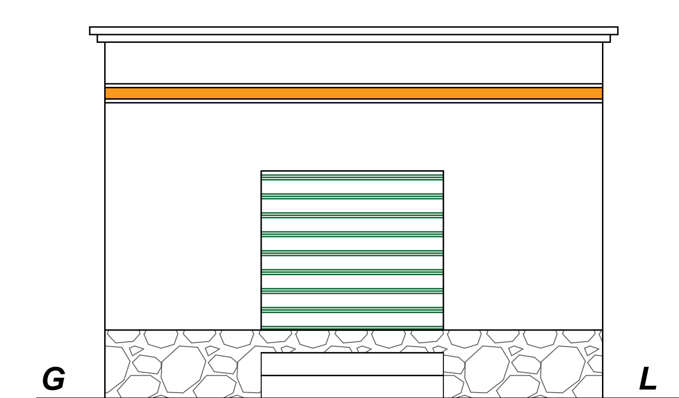
ELEVATION
