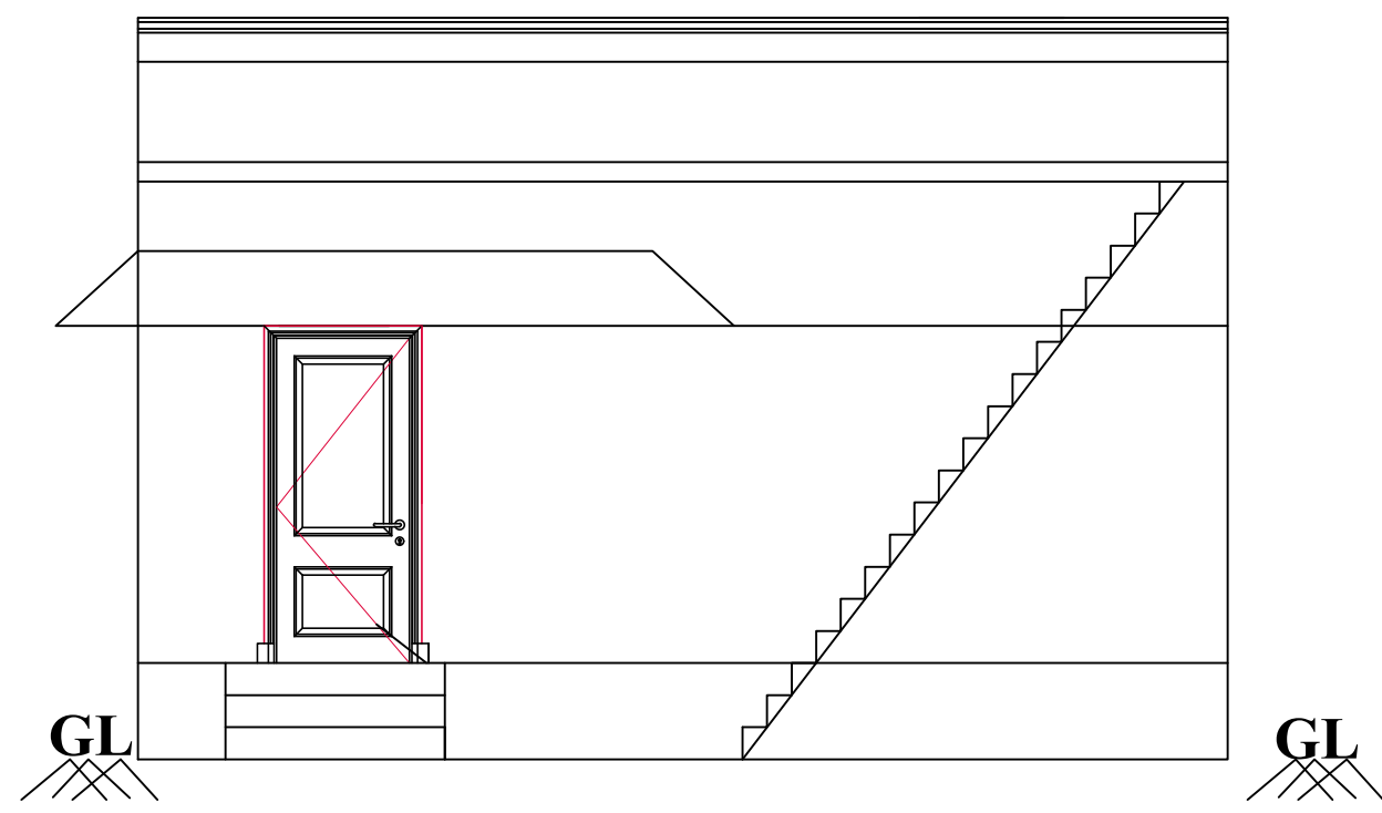
ELEVATION
