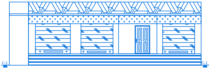
ELEVATION
