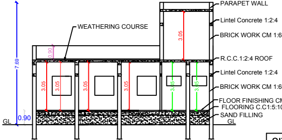
SECTION ON - AZ
