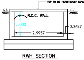
R.W.H. SECTION
