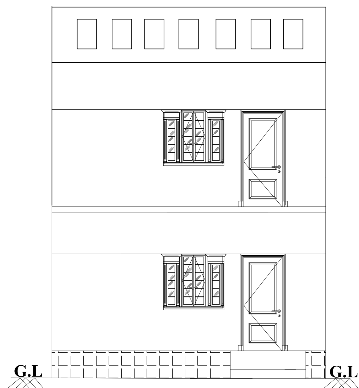
ELEVATION
