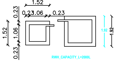
RWH_CAPACITY_L=2000L
