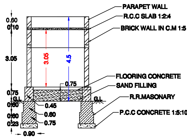
SECTION 'AB'
