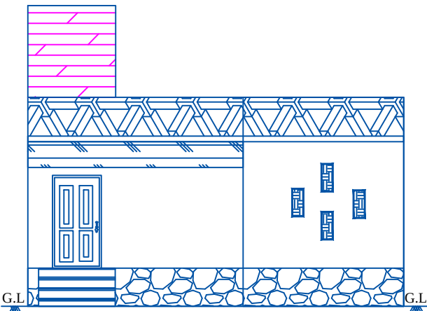
ELEVATION
