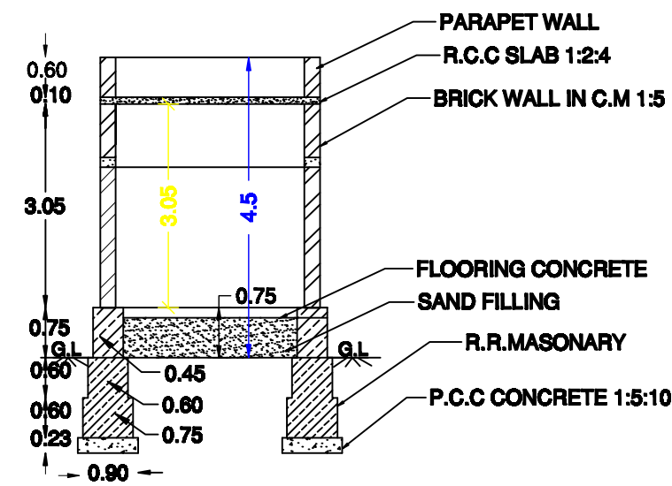
SECTION 'AB'
