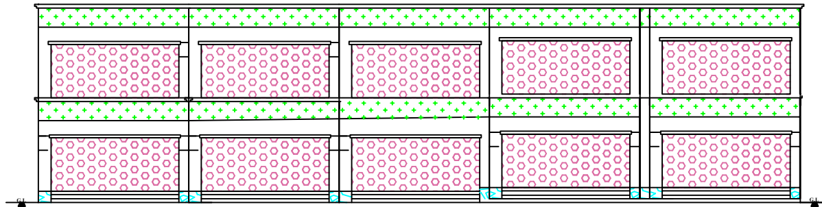
ELEVATION
