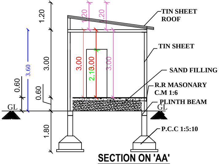
CHELLAPPA HOUSE 19'6"(6.00)
