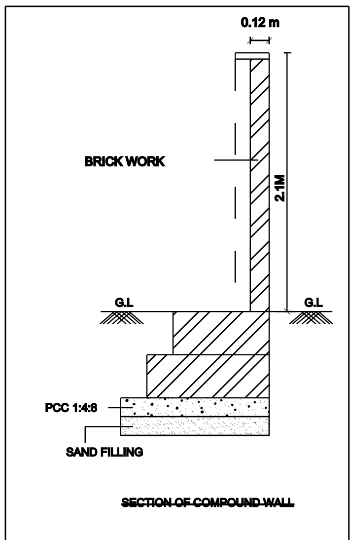
SURVEY NO : 384/1B1 LAND
