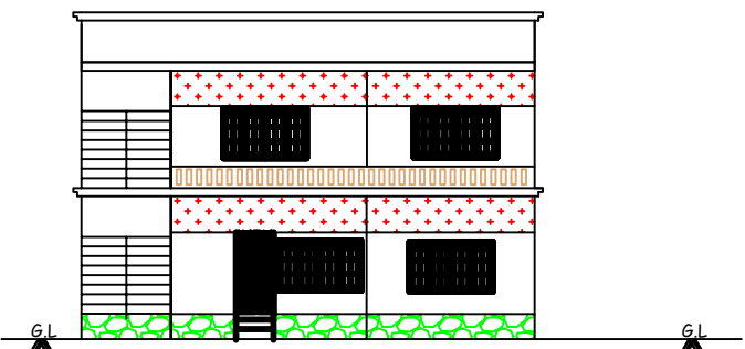
ELEVATION
