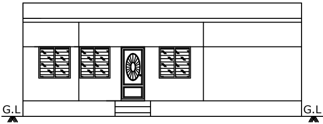
ELEVATION
