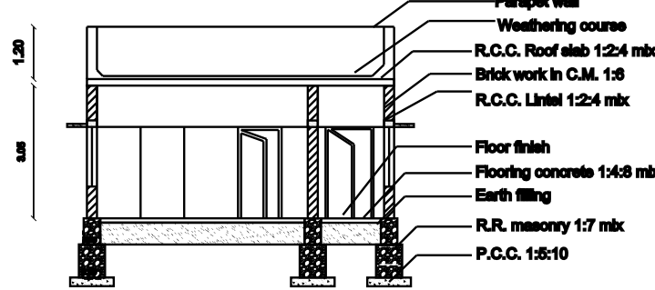
SECTION A-B
