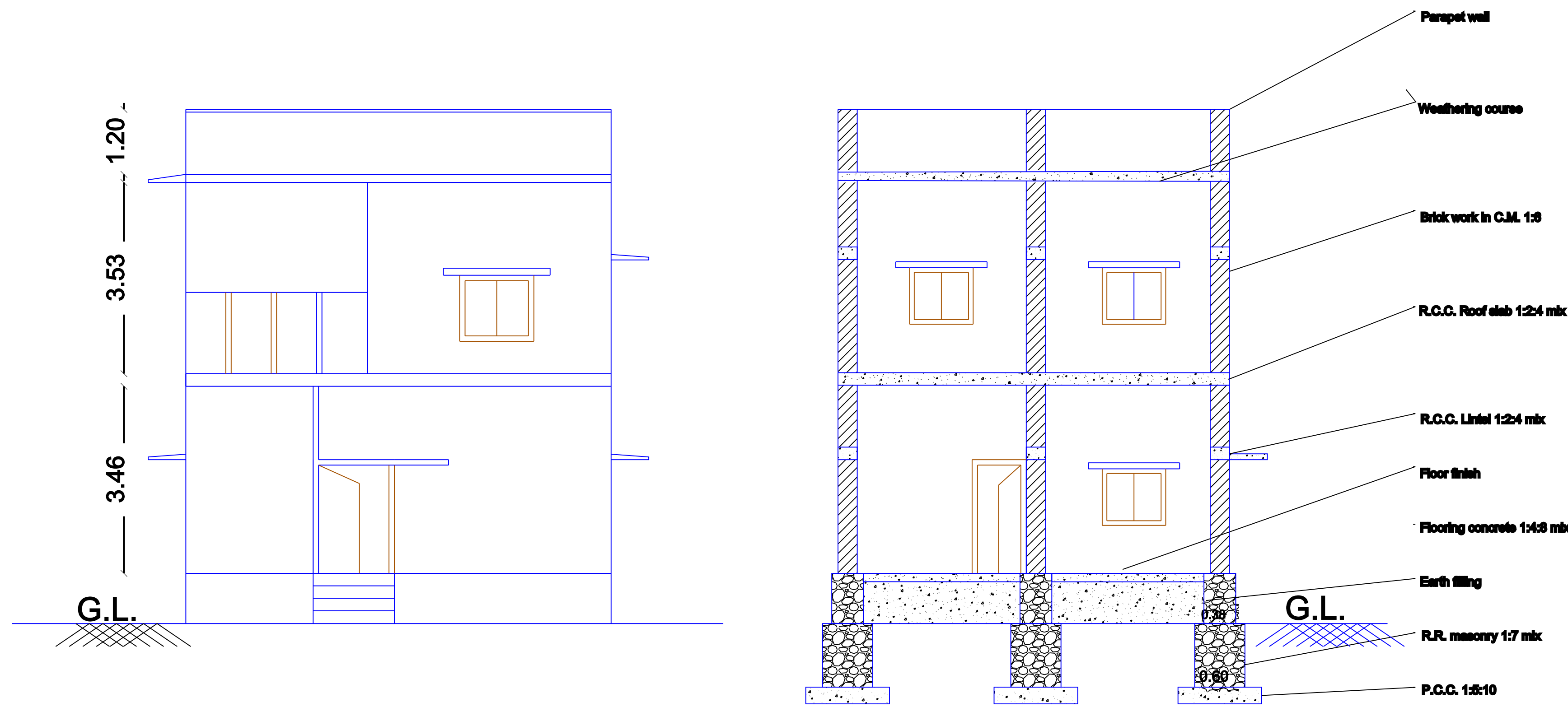
ELEVATION
