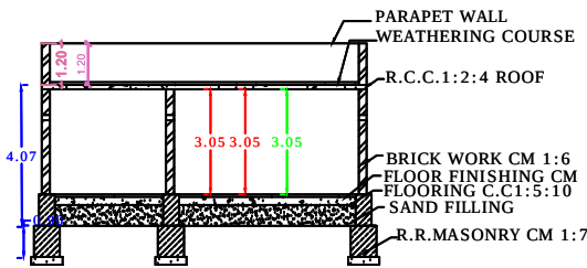
SECTOIN ON SV
