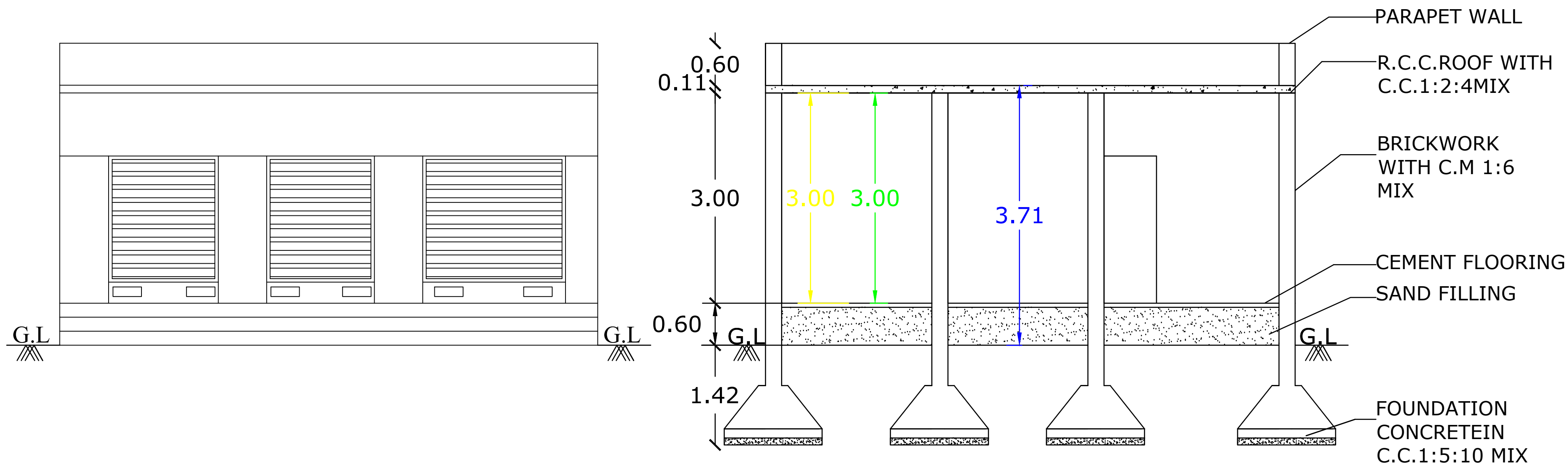
ELEVATION
