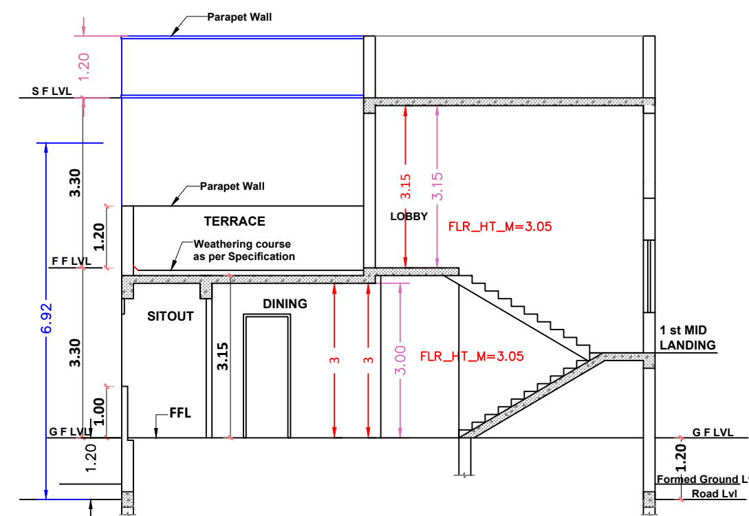
SECTION ON : 1-1
