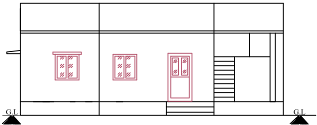
ELEVATION
