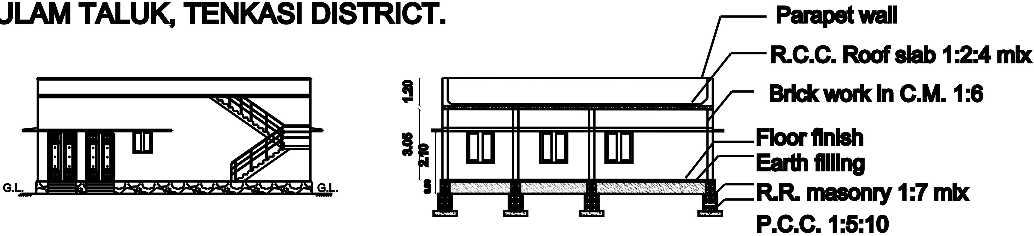
ELEVATION
