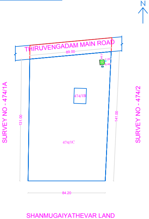
SITE PLAN (Scale 1:600)
