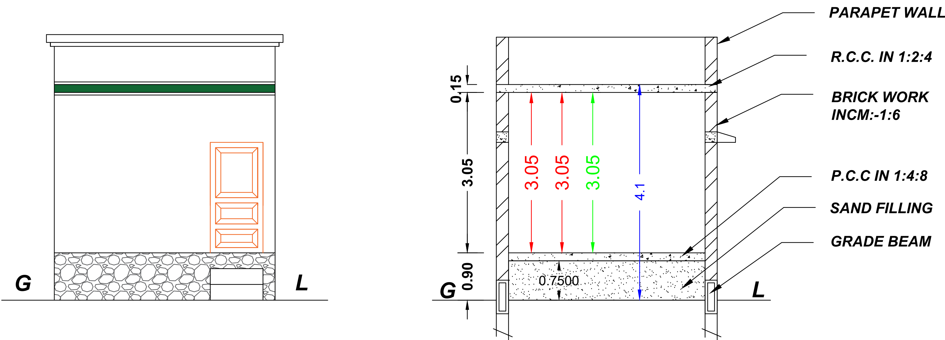
ELEVATION
