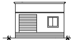
ELEVATION
