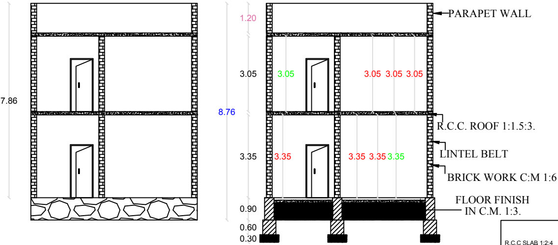
ELEVATION
