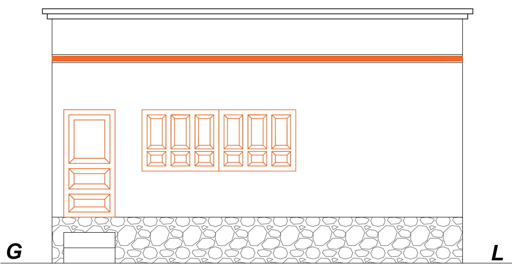
ELEVATION
