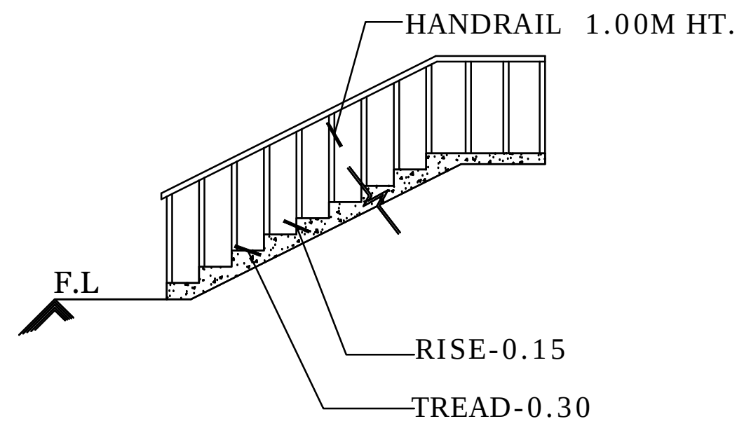
STAIRCASE DETAIL (N.T.S)
