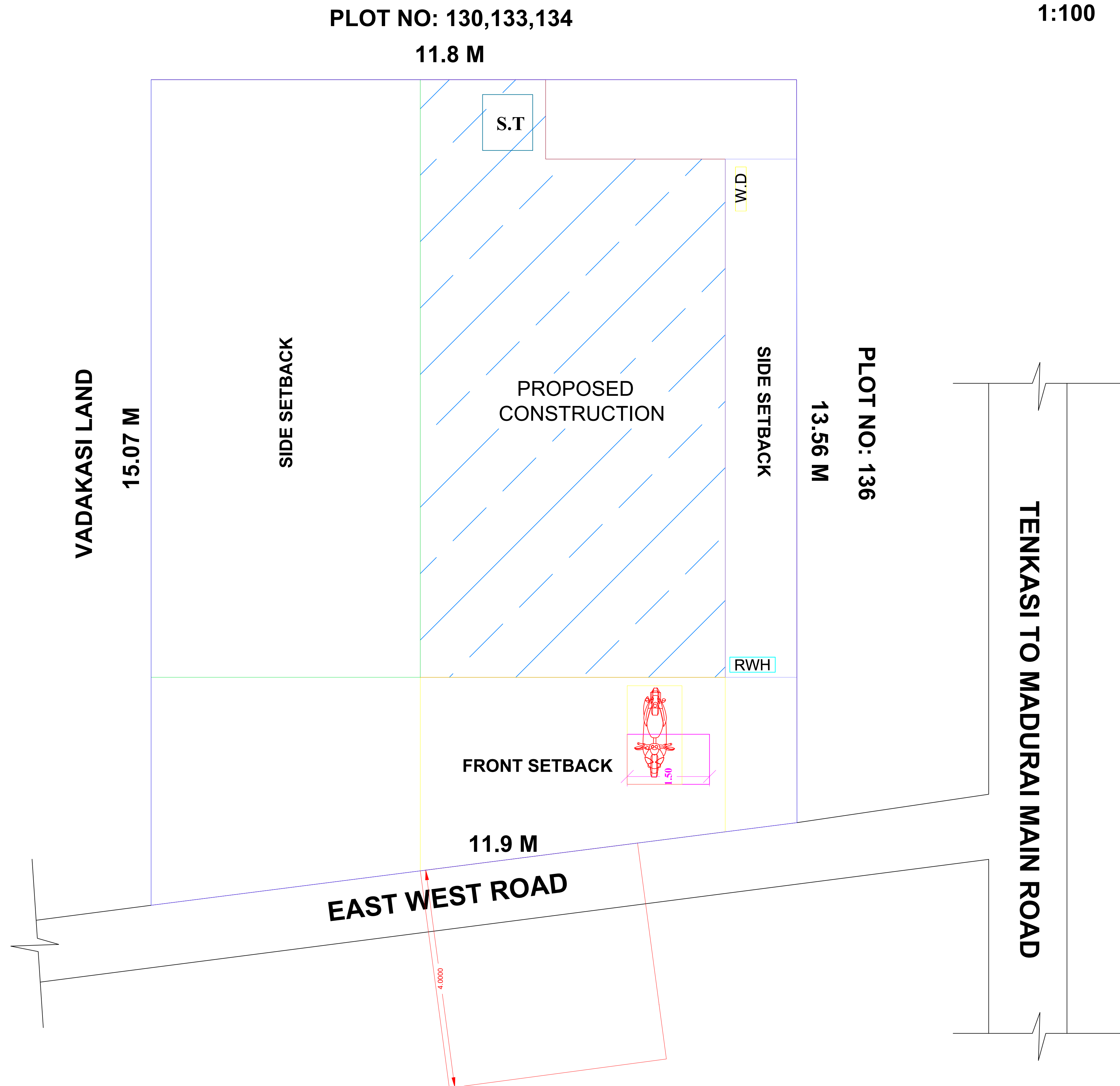
SITE PLAN 1:100
