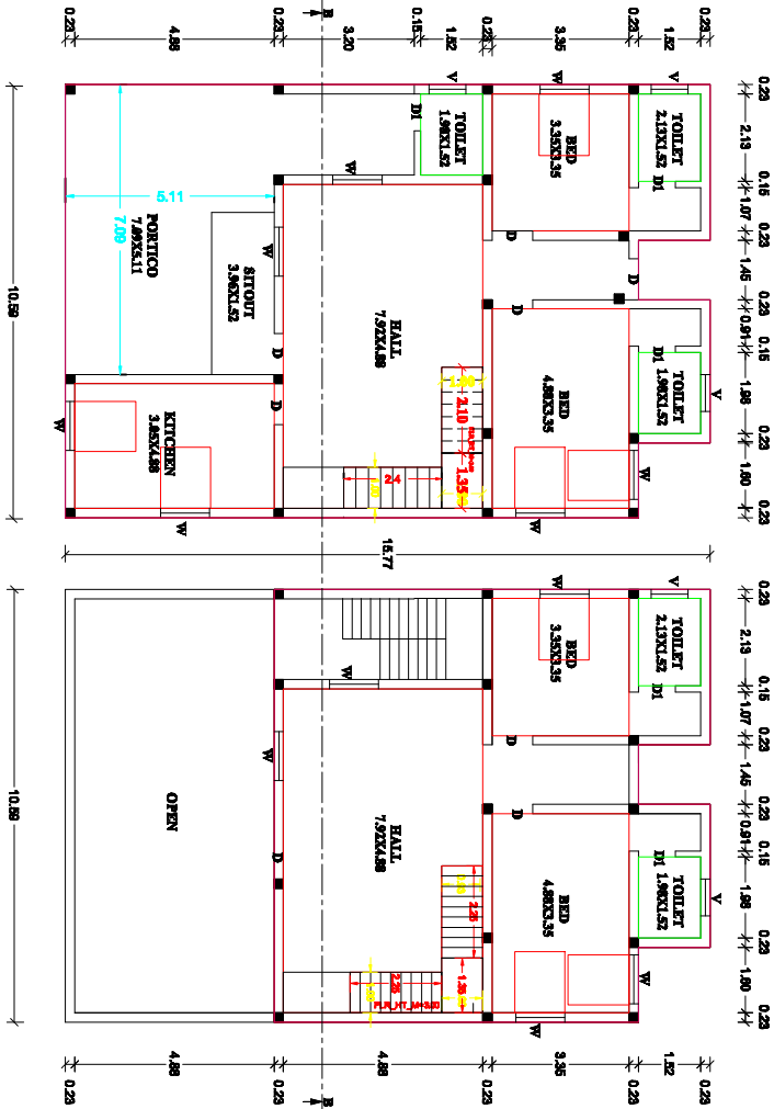
PRO. G.F. PLAN
