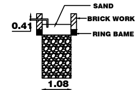
SECTION ON OP
