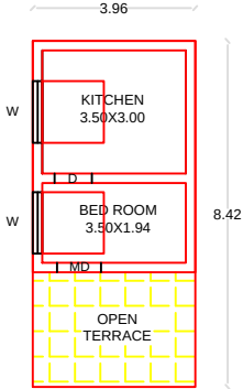
PRO FF PLAN
