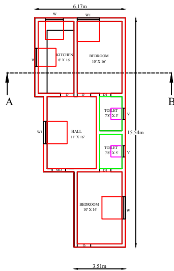
UND FLOOR PLAN
