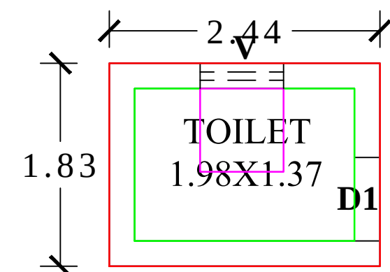
TOILET PLAN
