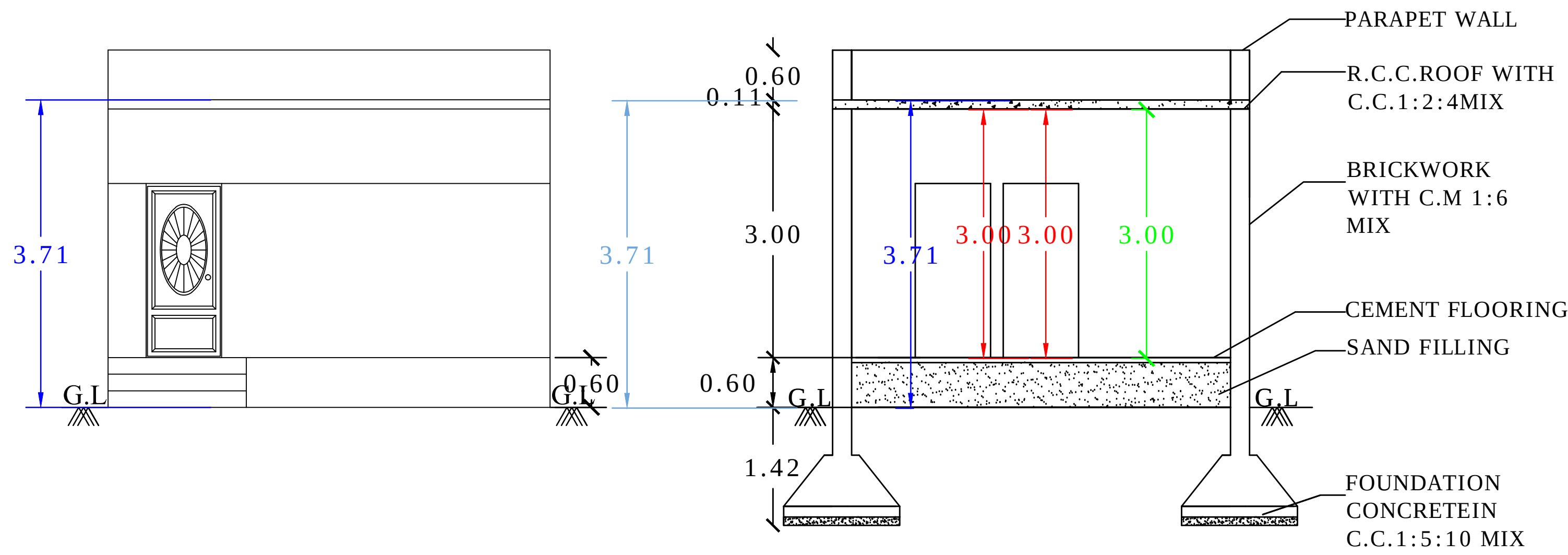
ELEVATION
