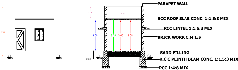
ELEVATION
