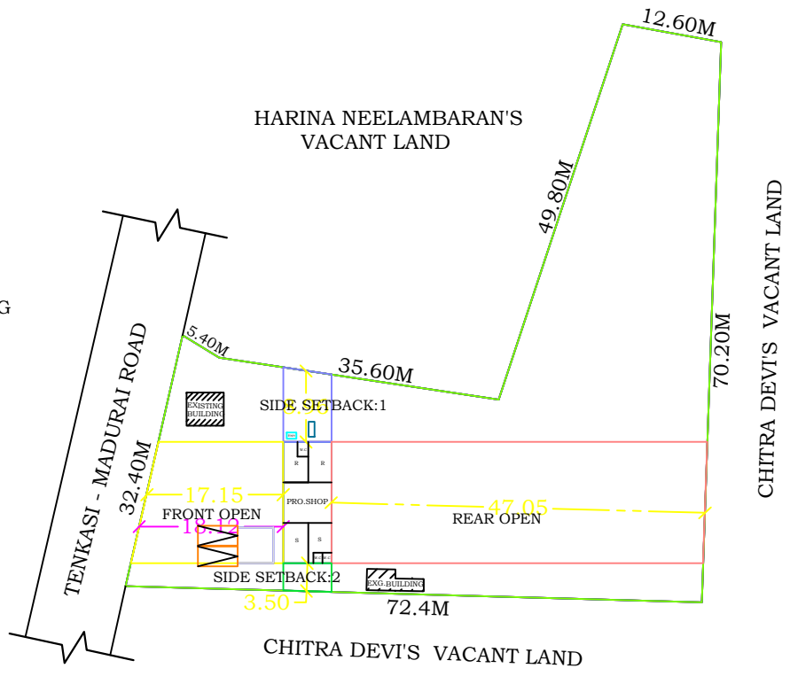
SITE PLAN SCALE-1:800
