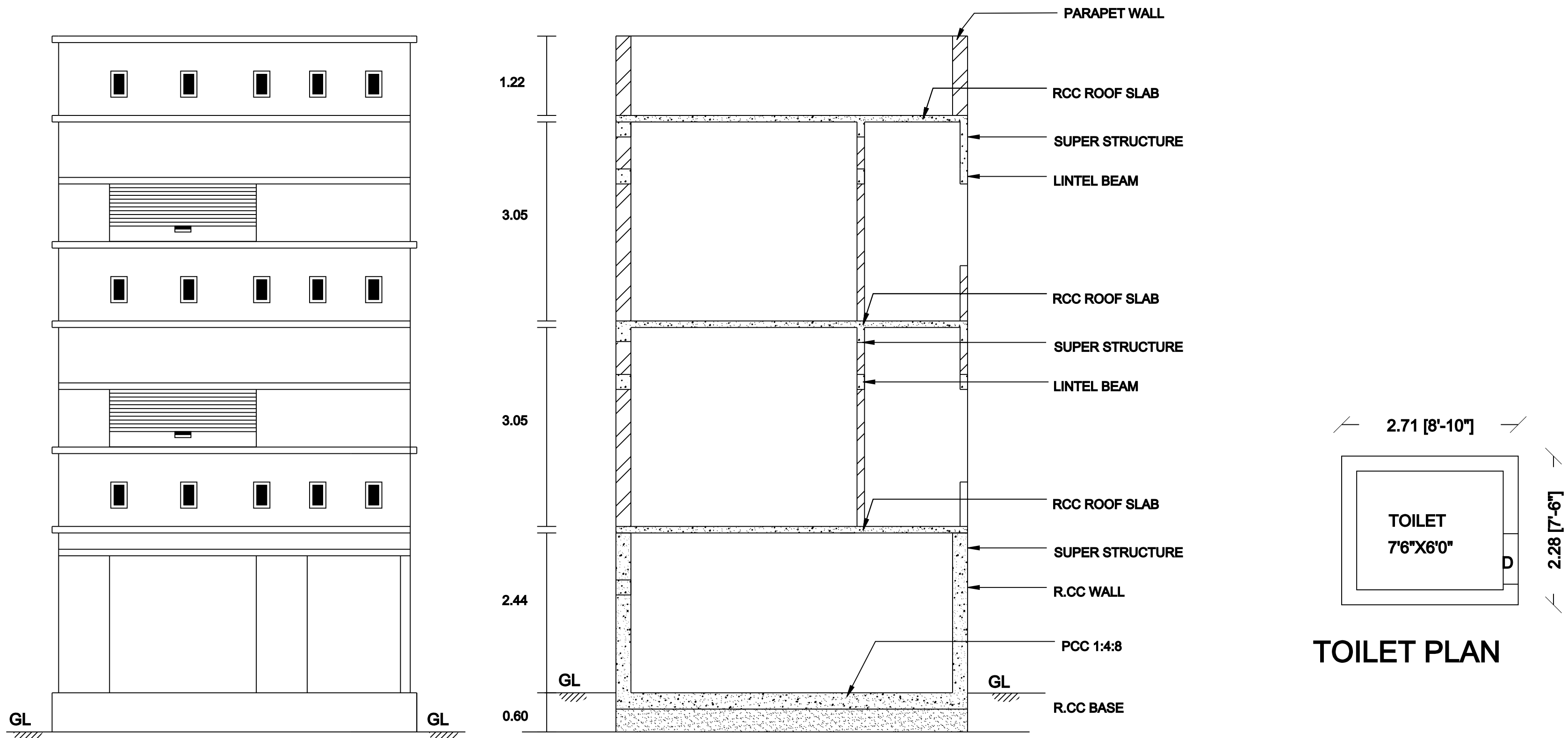
ELEVATION
