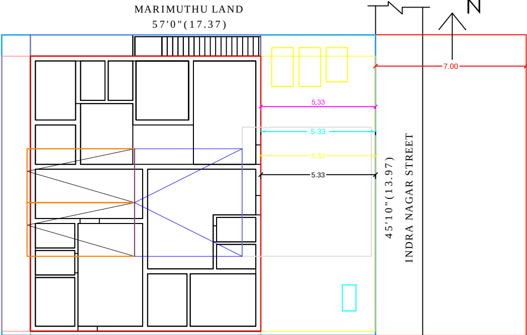
JEGANATHAN LAND SITE PLAN SCALE 1:100
