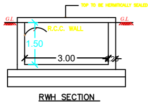
R.W.H. SECTION
