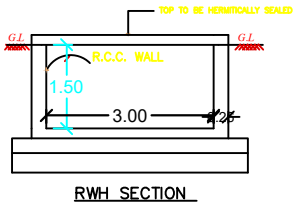
R.W.H. SECTION
