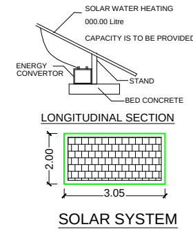
LONGITUDINAL SECTION
