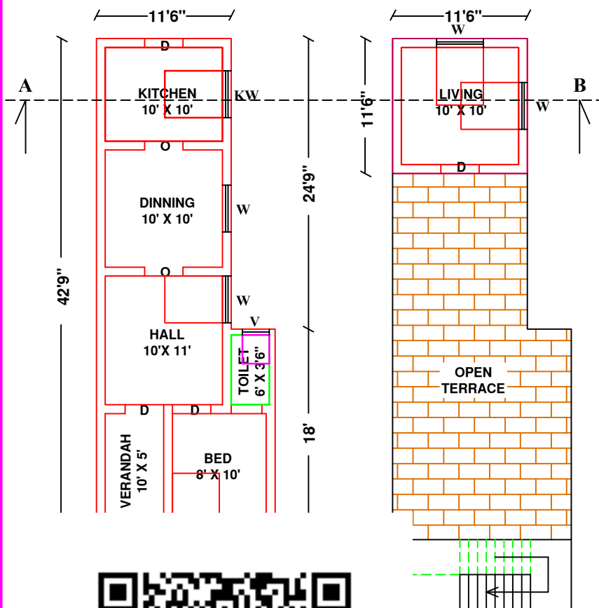
PRO. "FF" PLAN
