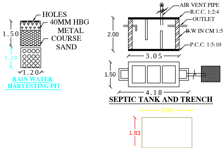
ELEVATION
