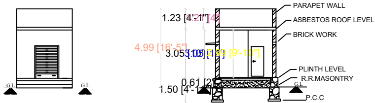
ELEVATION
