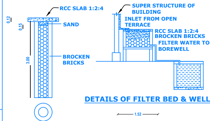
PERCOLATIONN PIT
