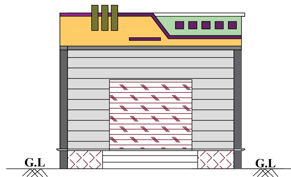
ELEVATION
