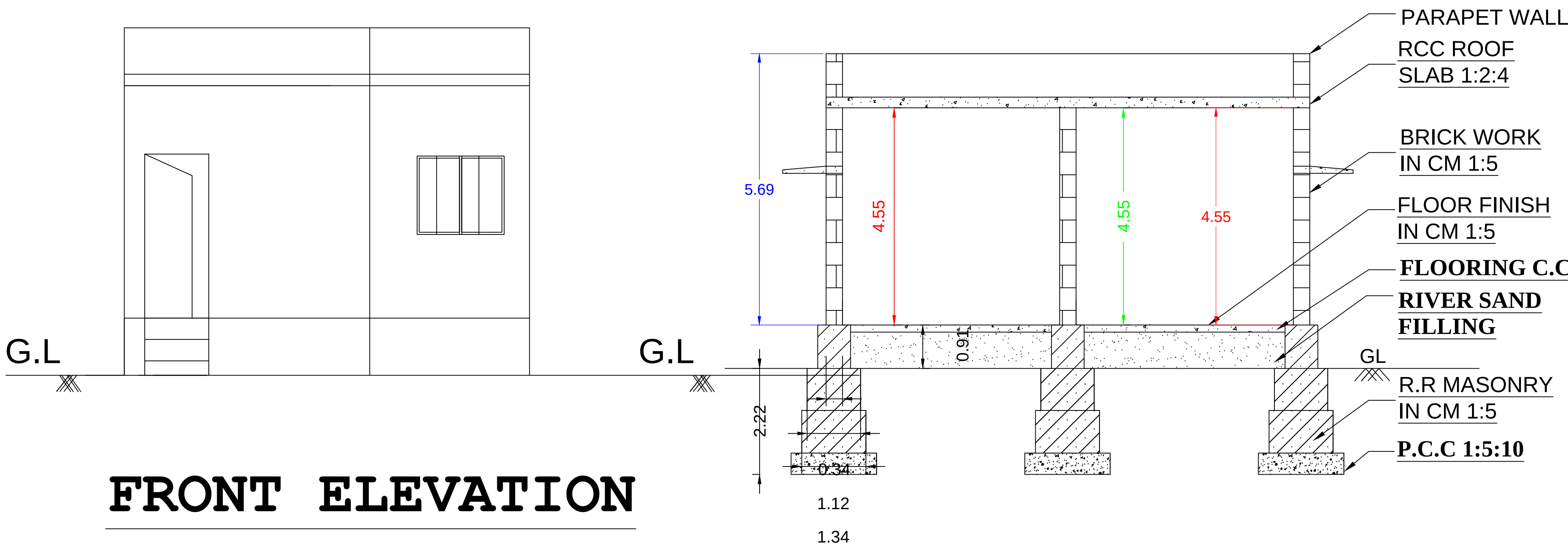
SECTION A-A
