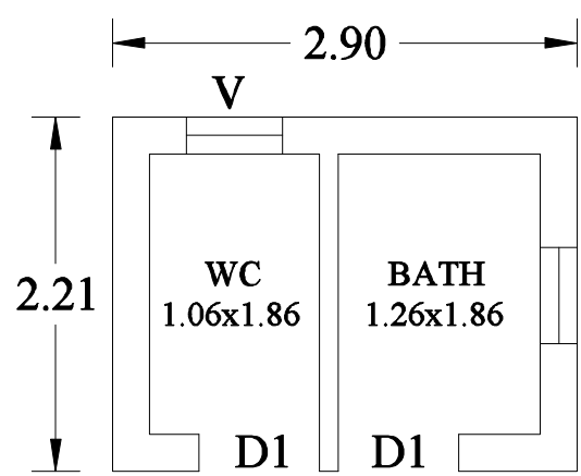
TOILET/BATH PLAN
