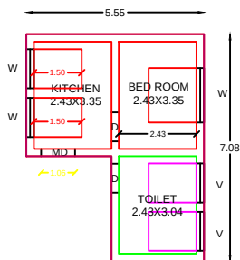
PRO G. FLOOR PLAN
